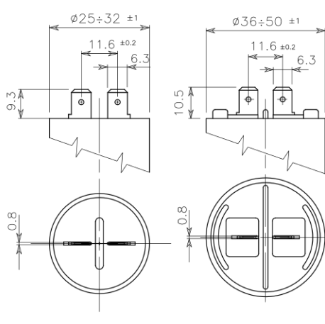
Fig. 2 Faston Semplice 6,3 x 0,8 mm Single tag 6.3 x 0.8 mm
