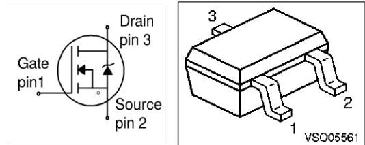
PG-SOT-323
