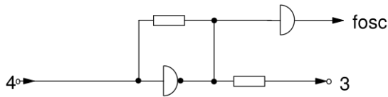
Fig. 4-6: X1, X2
