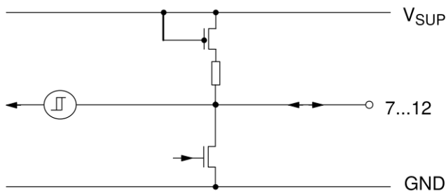
Fig. 4-8: IM bus
