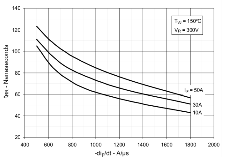
Fig. 24. Recover Time t_{RR} vs. -di_F/dt
