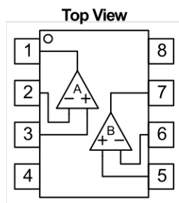
DIP8, DMP8, SSOP8 Package
