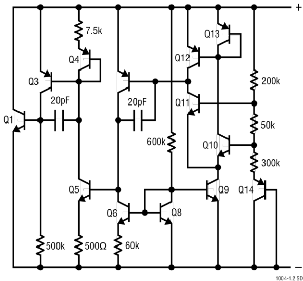
LT1004-1.2
