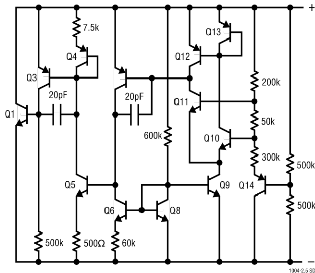
LT1004-2.5
