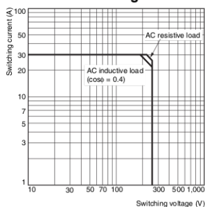
G7L-1A-T (TJ) (TUBJ) G7L-1A-B (BJ) (BUB) (BUBJ) Maximum Switching Power
