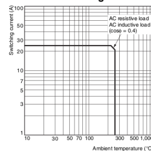
G7L-2A-T (TJ) (TUBJ) G7L-2A-B (BJ) (BUB) (BUBJ) Maximum Switching Power
