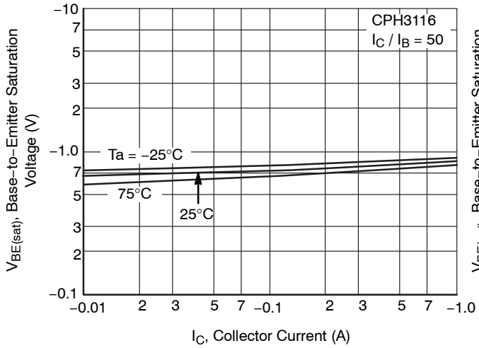
Figure 16. V_{BE(sat)} - I_C
