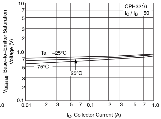
Figure 17. V_{BE(sat)} - I_C
