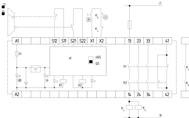
Abb. 4 a) Ansteuerlogik
