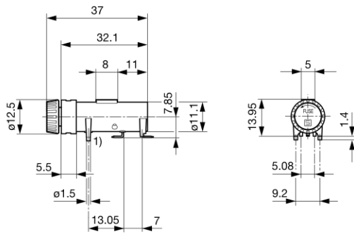
Variante 3101.0076 1) Befestigungsstifte
