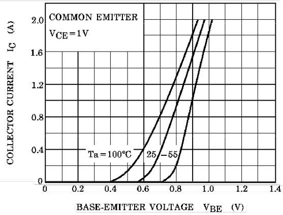
I C - V BE
