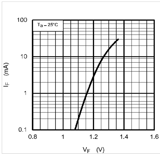
Fig. 13.1.3 I F - V F
