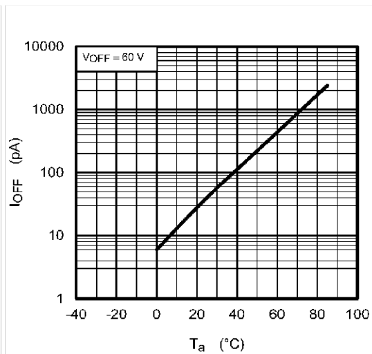
Fig. 13.1.10 I_{OFF} - T_a
