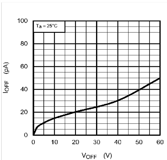
Fig. 13.1.9 I_{OFF} - V_{OFF}
