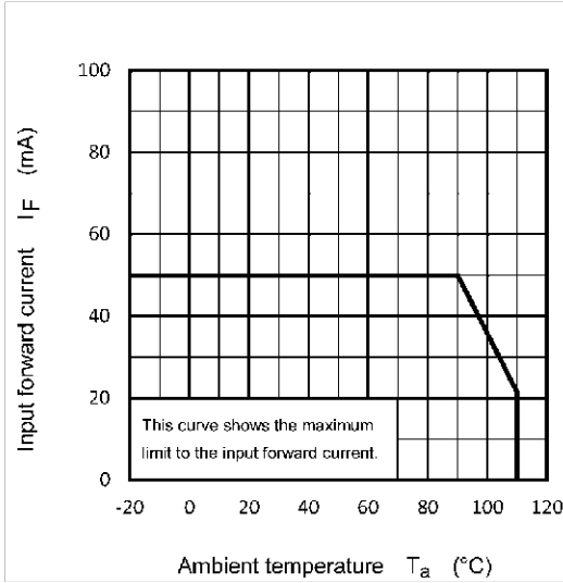
Fig. 11.1 I_F - T_a
