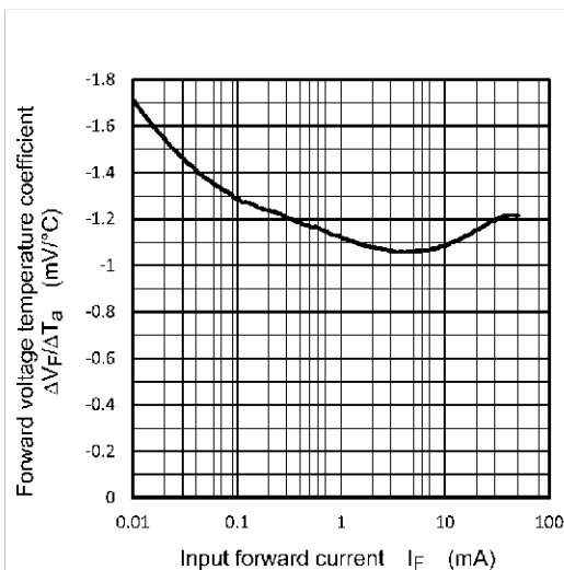
Fig. 11.5 \Delta V_F / \Delta T_a - I_F
