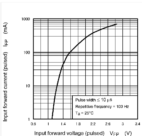
Fig. 11.6 I_{FP} - V_{FP}
