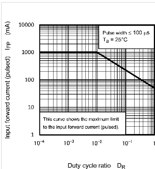
Fig. 11.3 I_{FP} - D_R
