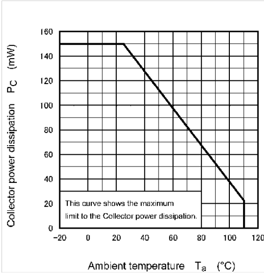
Fig. 11.2 P_C - T_a
