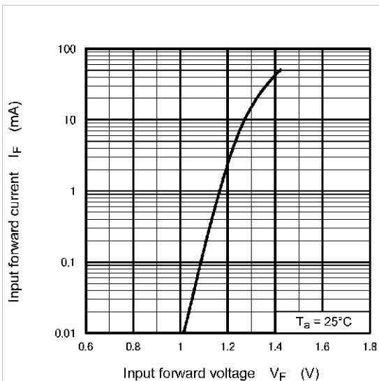
Fig. 11.4 I_F - V_F
