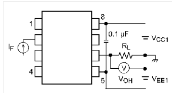
Fig. 13.1.3 V_{OH} Test Circuit
