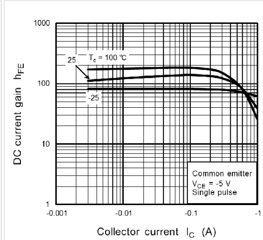
Fig. 7.2 h_{FE} - I_C
