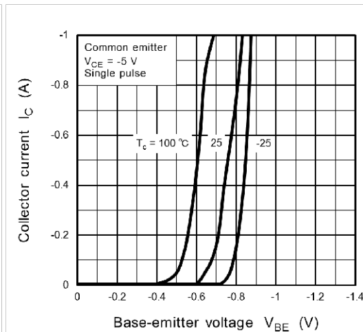
Fig. 7.4 I_C - V_{BE}
