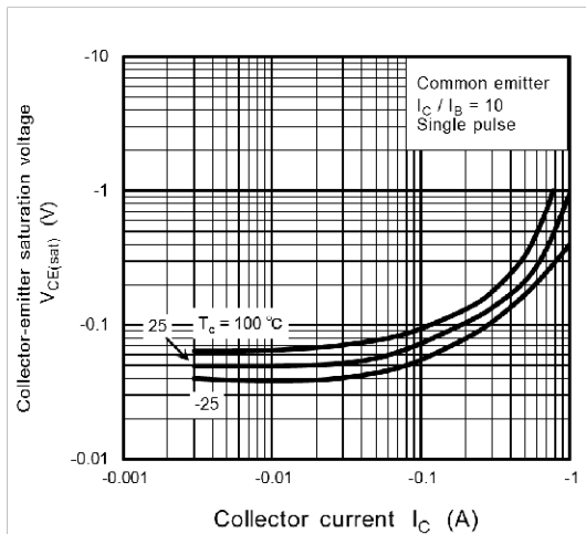
Fig. 7.3 V_{CE(sat)} - I_C
