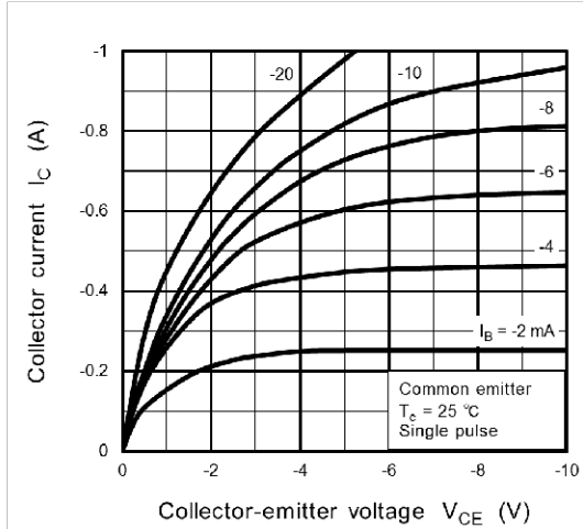
Fig. 7.1 I_C - V_{CE}
