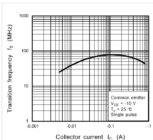
Fig. 7.5 f_T - I_C
