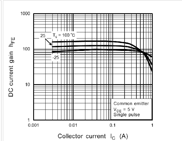
Fig. 7.2 hFE - IC
