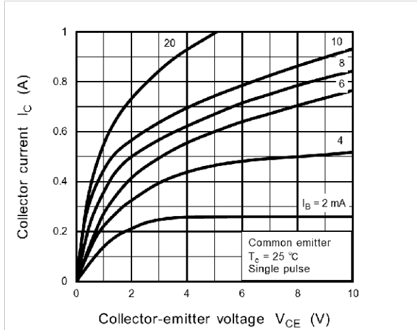
Fig. 7.1 IC - VCE
