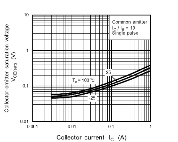
Fig. 7.3 VCE(sat) - IC
