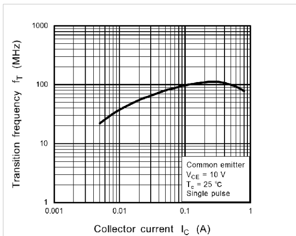
Fig. 7.5 fT - IC
