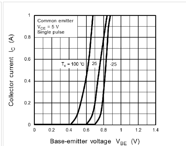
Fig. 7.4 IC - VBE
