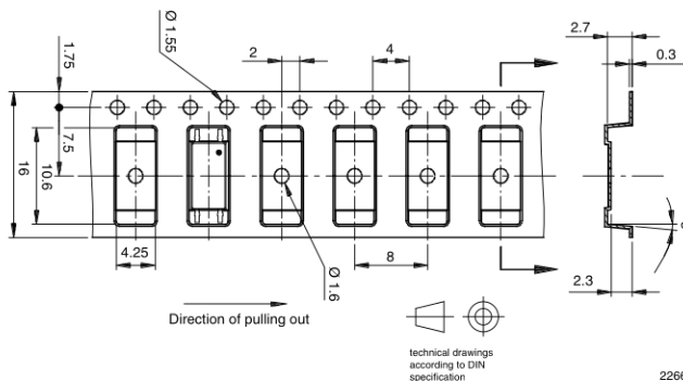
Fig. 20 - Tape Dimensions
